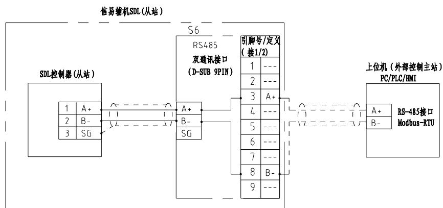
SDL RS-485通讯接线示意图
