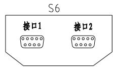
信易RS-485接口定义
