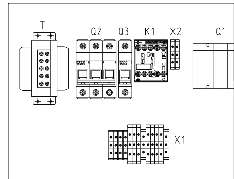
控制箱底板 Control Box Bottom Plate
