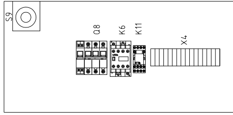
干燥箱1控制箱
