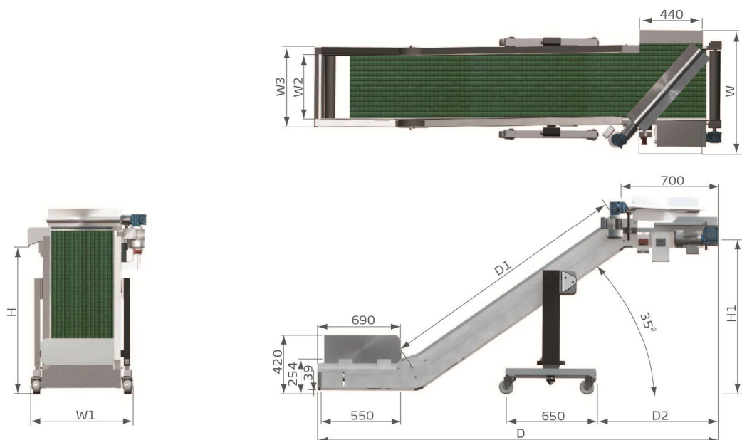
图 1-1: 外形尺寸图
