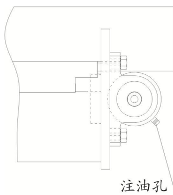
图 6-2: 轴承润滑图
