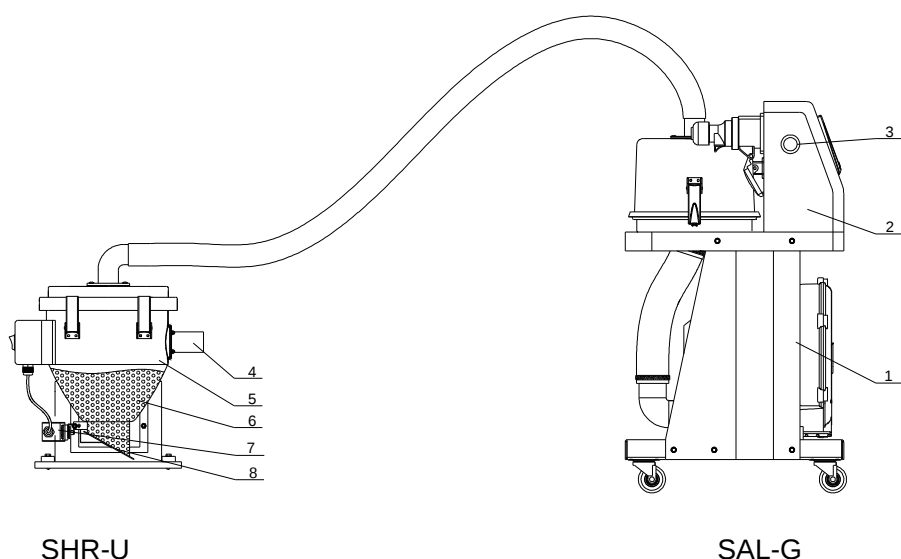
图 2-1: 工作原理图 1
