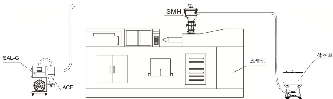
图 3-5: 选配 ACF 安装示意图
