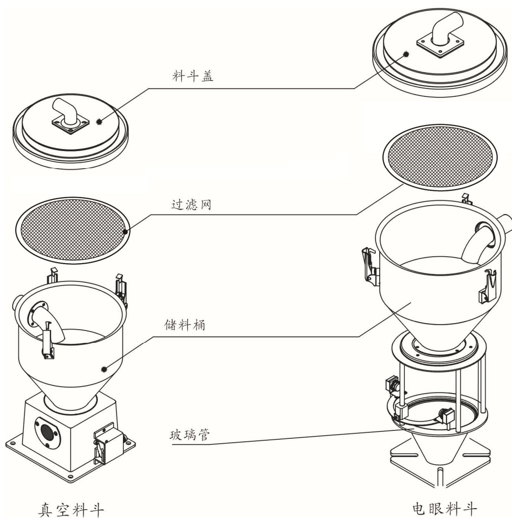
图 6-1: 料斗清洁图
