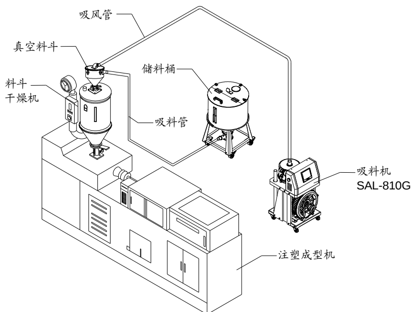
图 3-2: 安装示意图 2
