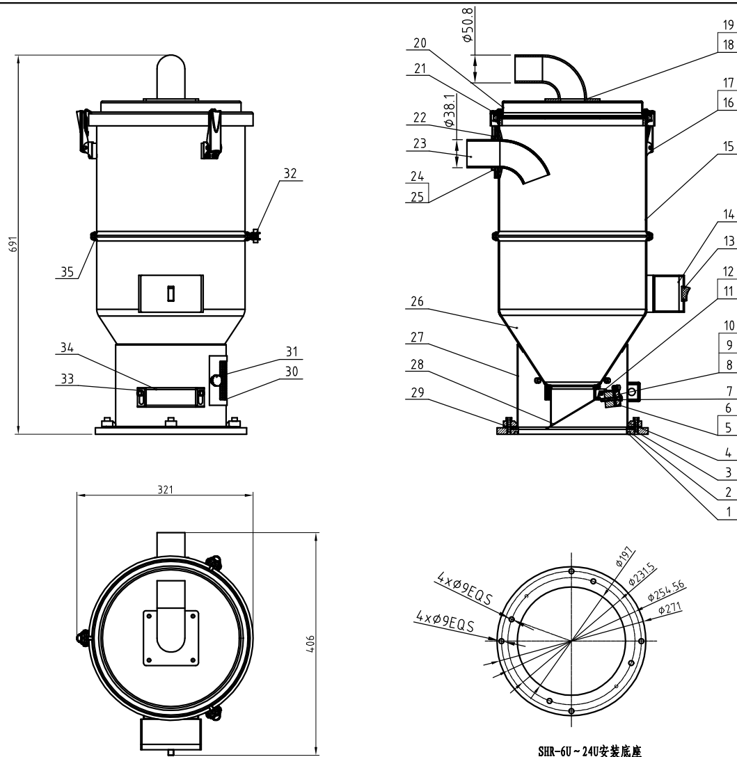
SHR-6U ~ 24U安装底座
