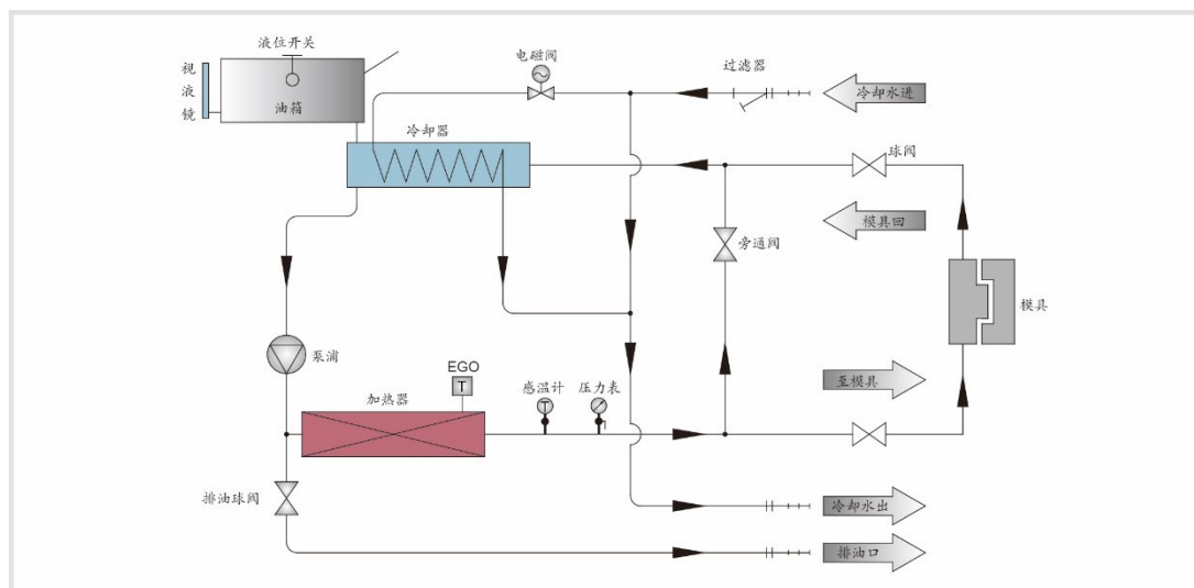
图 2-1: 工作原理图
