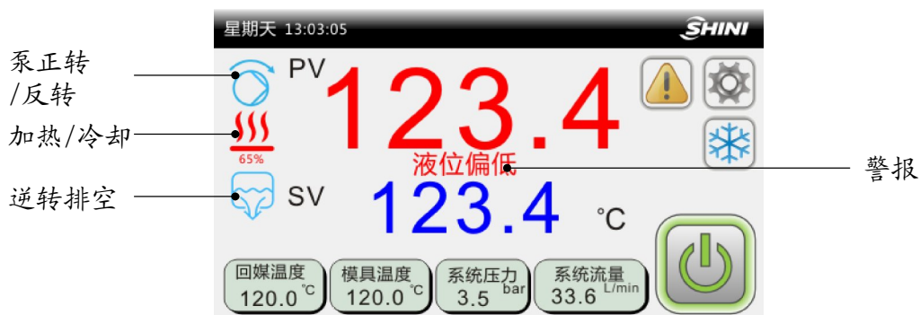
图 4-3: 运行画面
