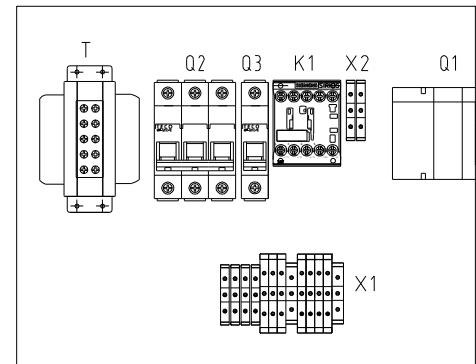
控制箱底板
