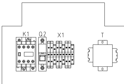
控制箱电器安装板
