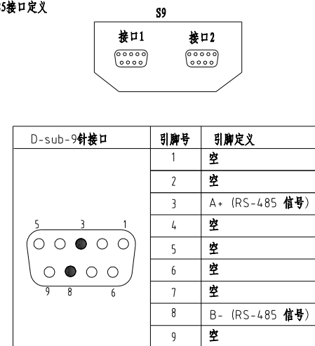
信易RS-485接口定义
