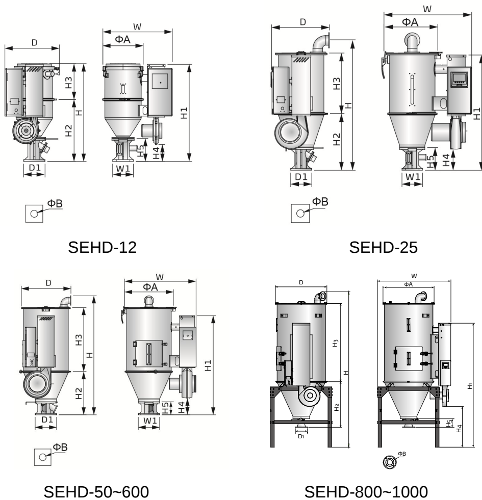
图 1-1: 外形尺寸图
