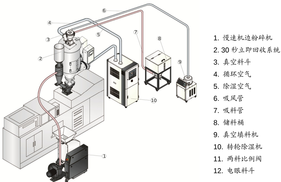
图 3-1: 直接安装型
