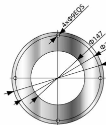
SHR-3U-S 安装底座
