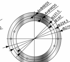
SHR-6U-S~SHR-24U-S 安装底座
