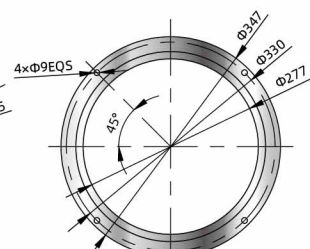
SHR-36U-S~SHR-96U-S 安装底座
