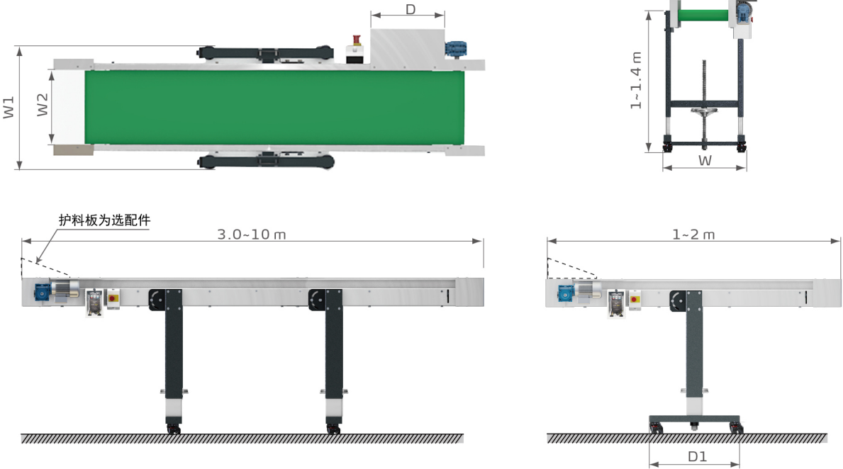
PNL系列外形尺寸图
