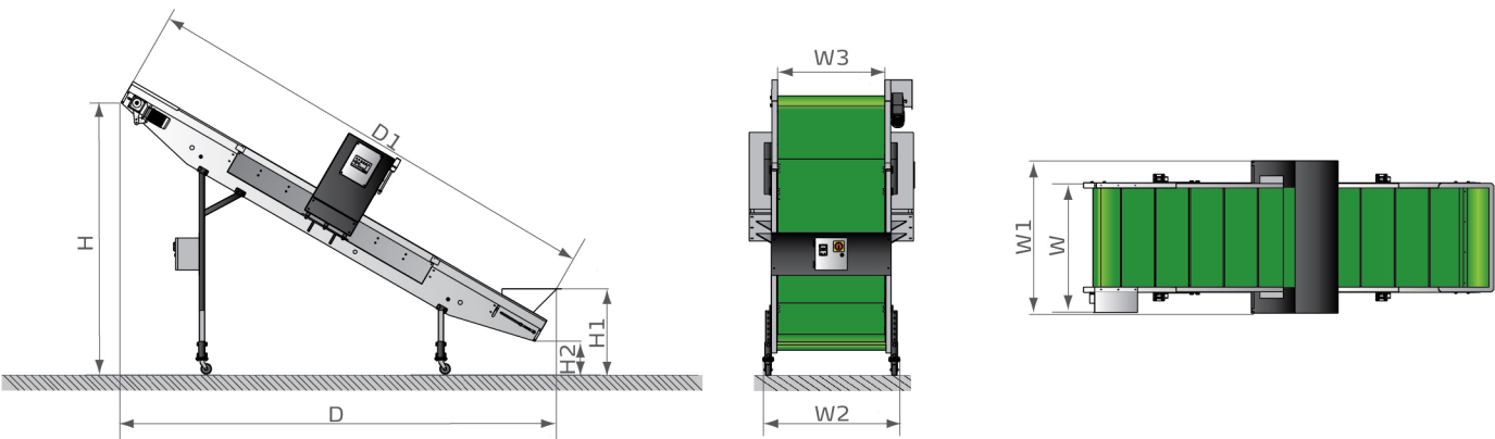
PNL-MS系列外形尺寸图
