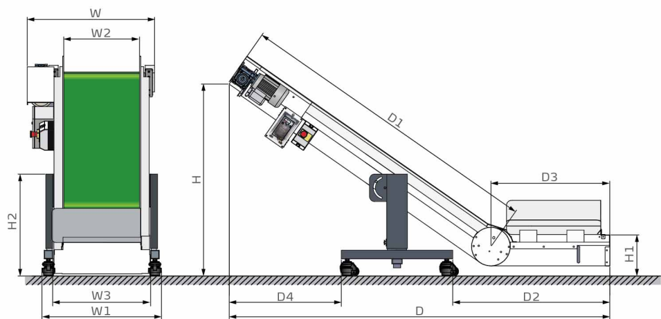
CB系列外形尺寸图
