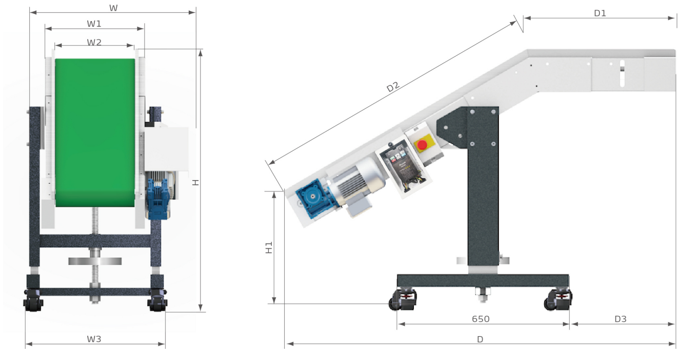
SV系列外形尺寸图
