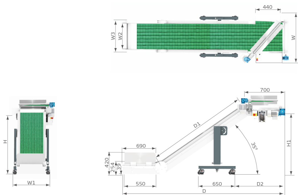
CBD 系列外形尺寸图
