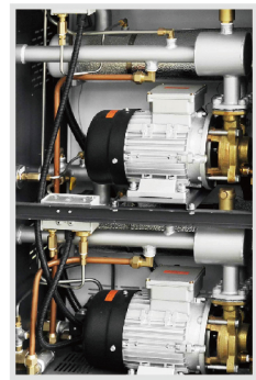
内部结构图
