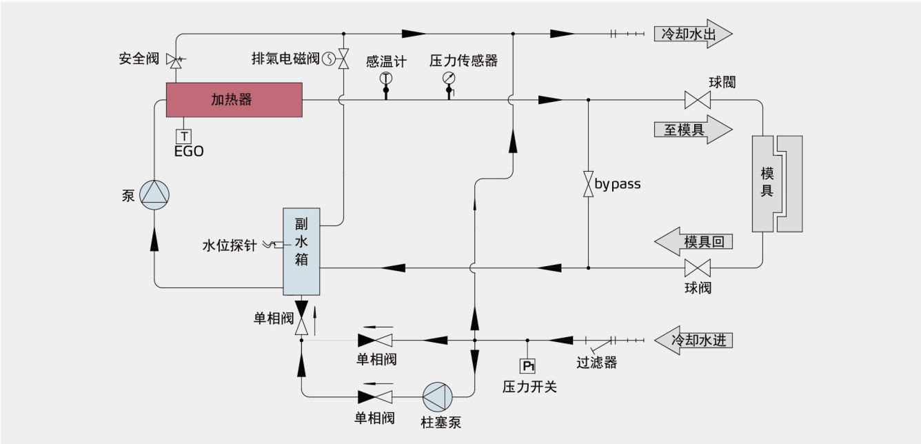
STM-DPW系统流程图
