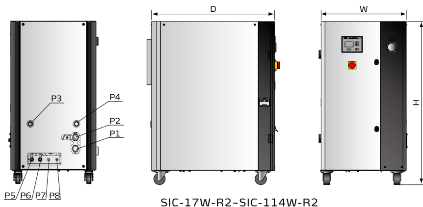
SIC-17W-R2~SIC-114W-R2 尺寸
