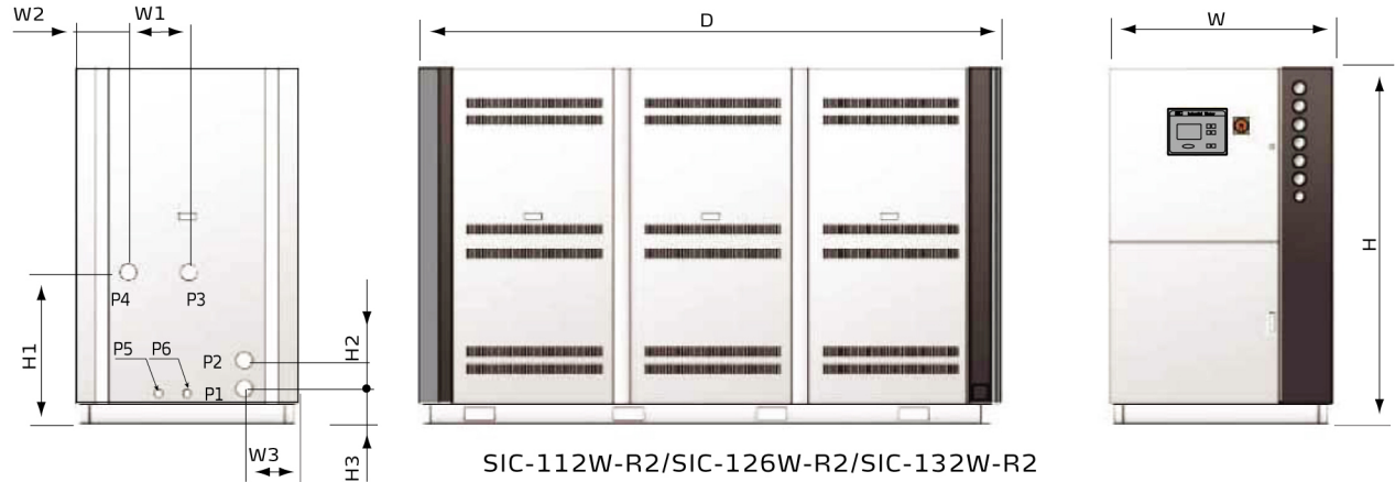
SIC-112W-R2/SIC-126W-R2/SIC-132W-R2 尺寸
