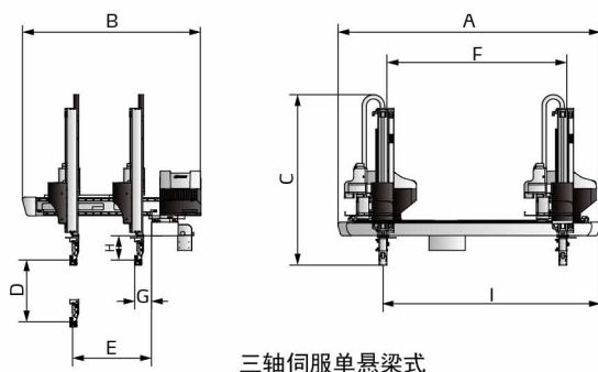
三轴伺服单悬梁式
